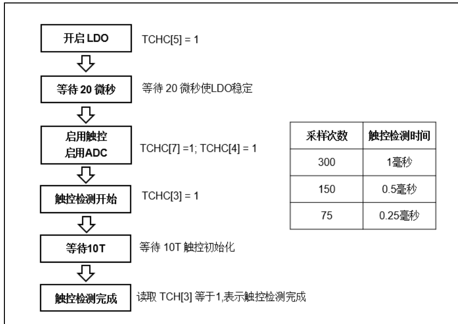
图 24：触控模式时序图
