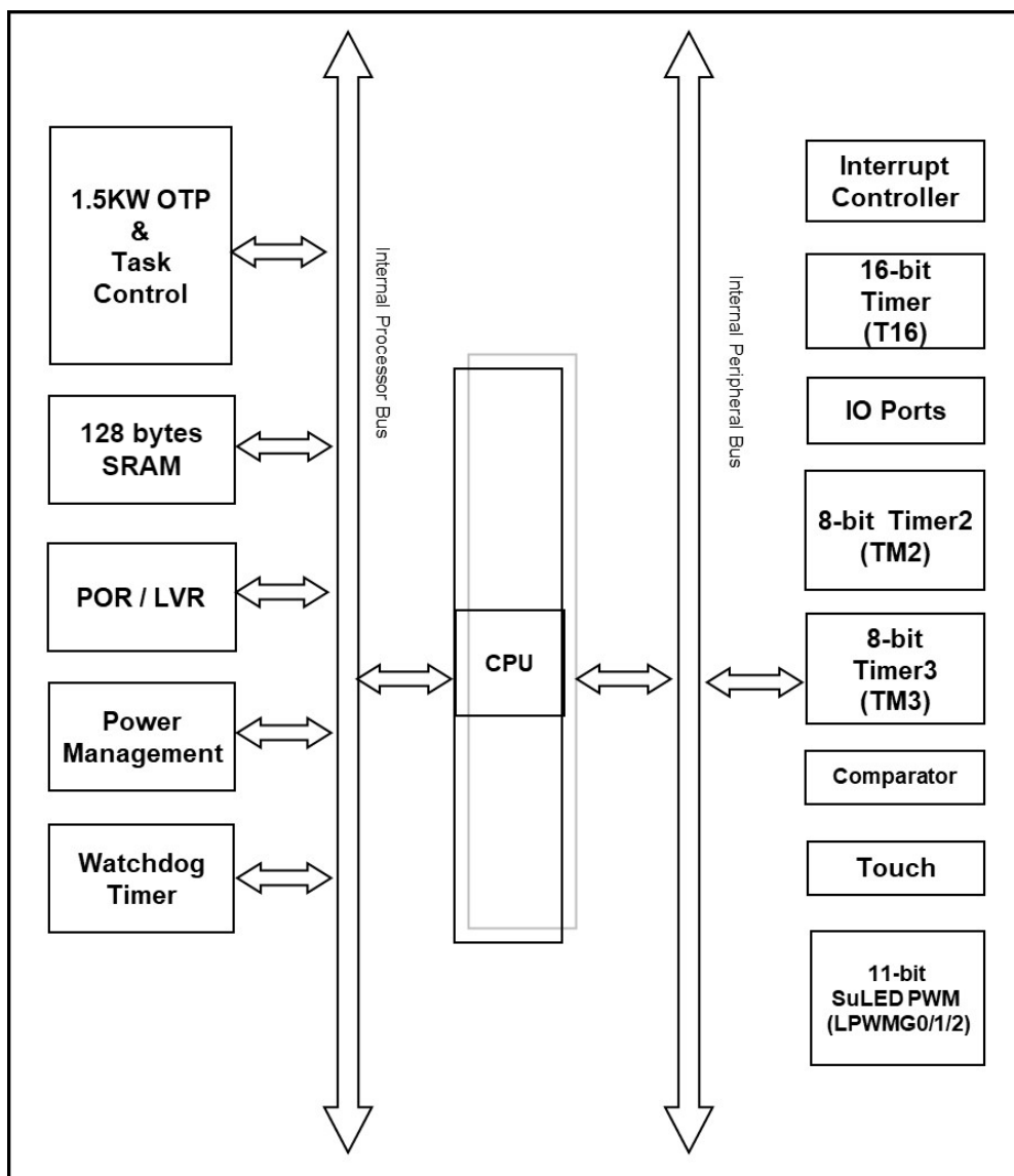
图 1: PMS160B 系统方框图
