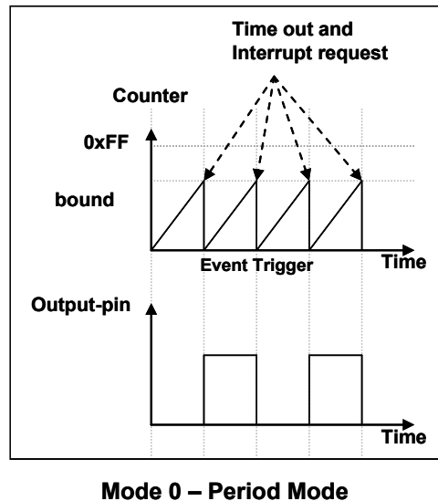
图 14: Timer2 周期模式的时序图
