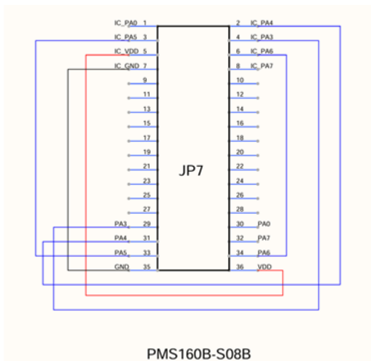
图 29：使用 P-003B 时，PMS160B-S08B JP7 跳线原理图
